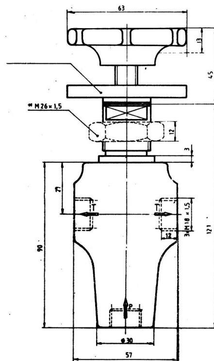
Fig.7.Supape reglabile ,cu roata de mana (M)
