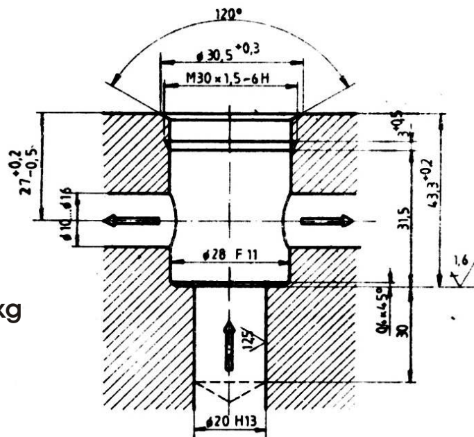
Fig.5 Locas pentru montajul supapei tip cartus
