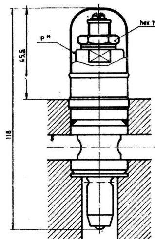
Fig.3 Supape reglabile cu surub, cu locas hexagonal (s)
