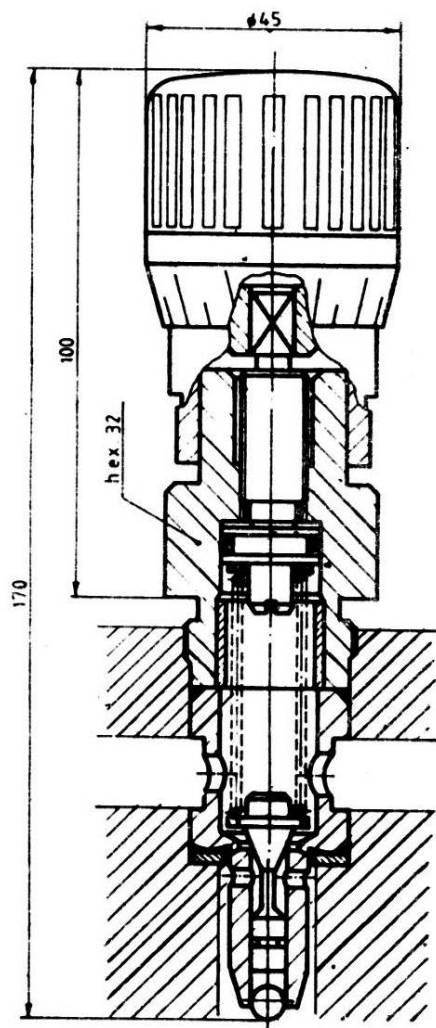
Fig.4 Supape reglabile cu cap gradat (G)
