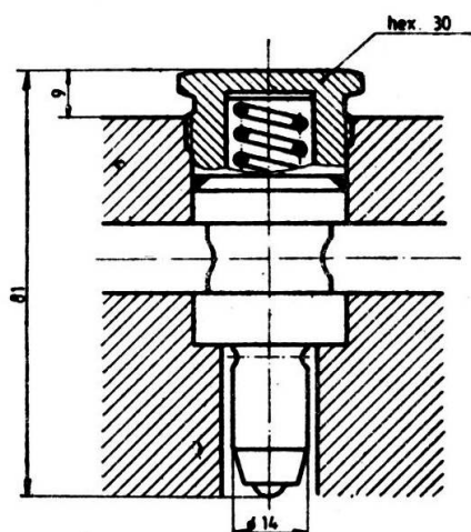
Fig.2 Supape cu reglaj fix
